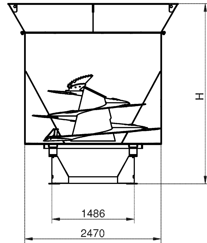
Schnitt A-A
